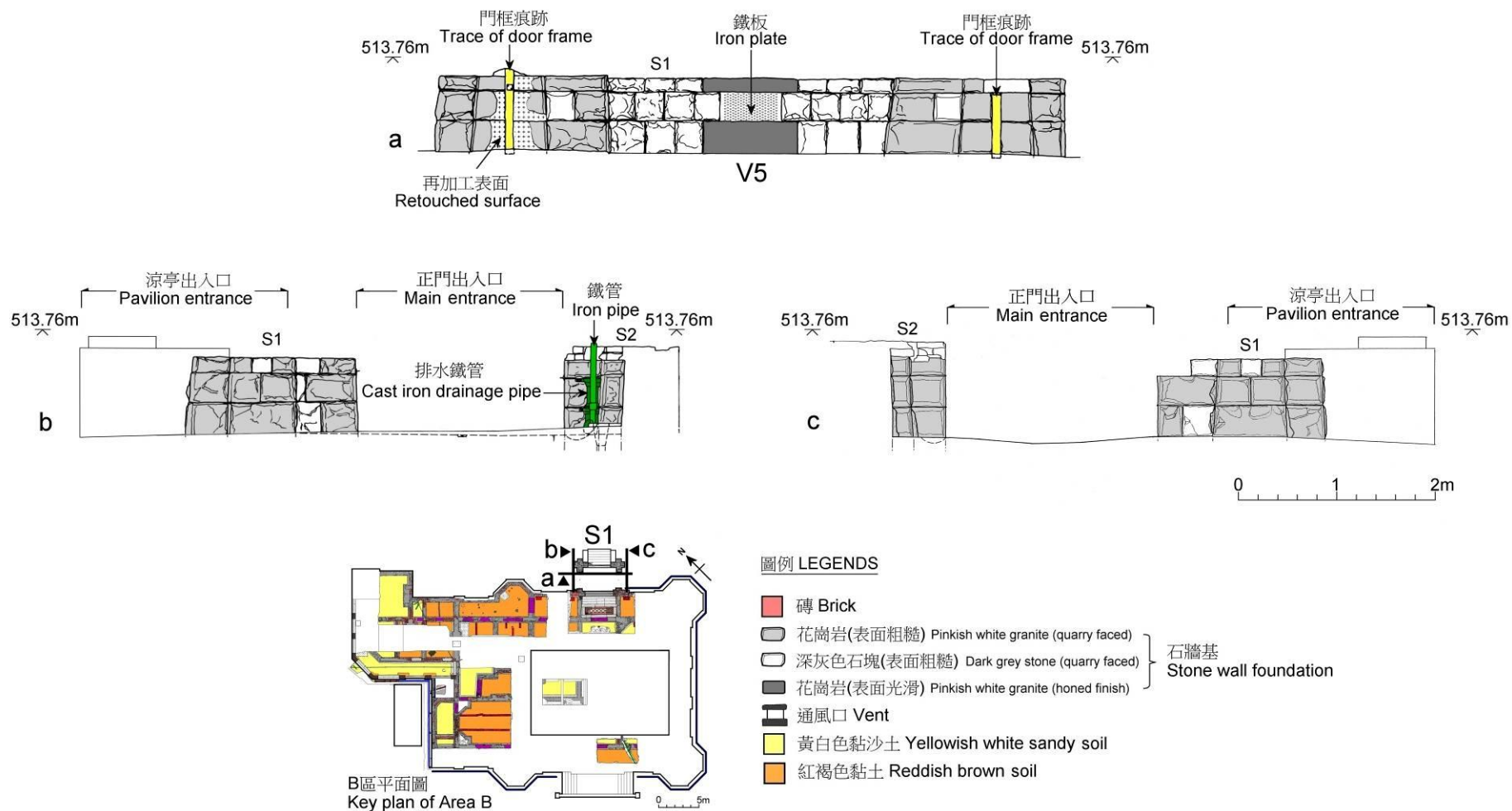
圖 33 石牆基 S1 側視圖 Fig 33 Side views of stone wall foundation S1
