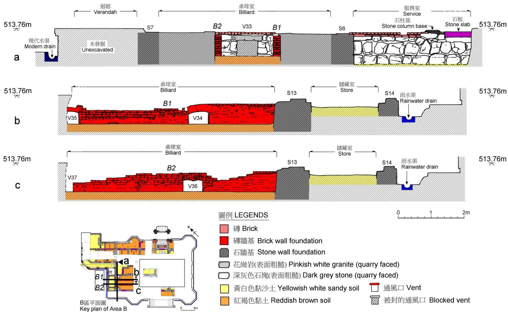
圖 50 磚牆基 B1 及 B2 側視圖 Fig 50 Side views of brick wall foundations B1 and B2
