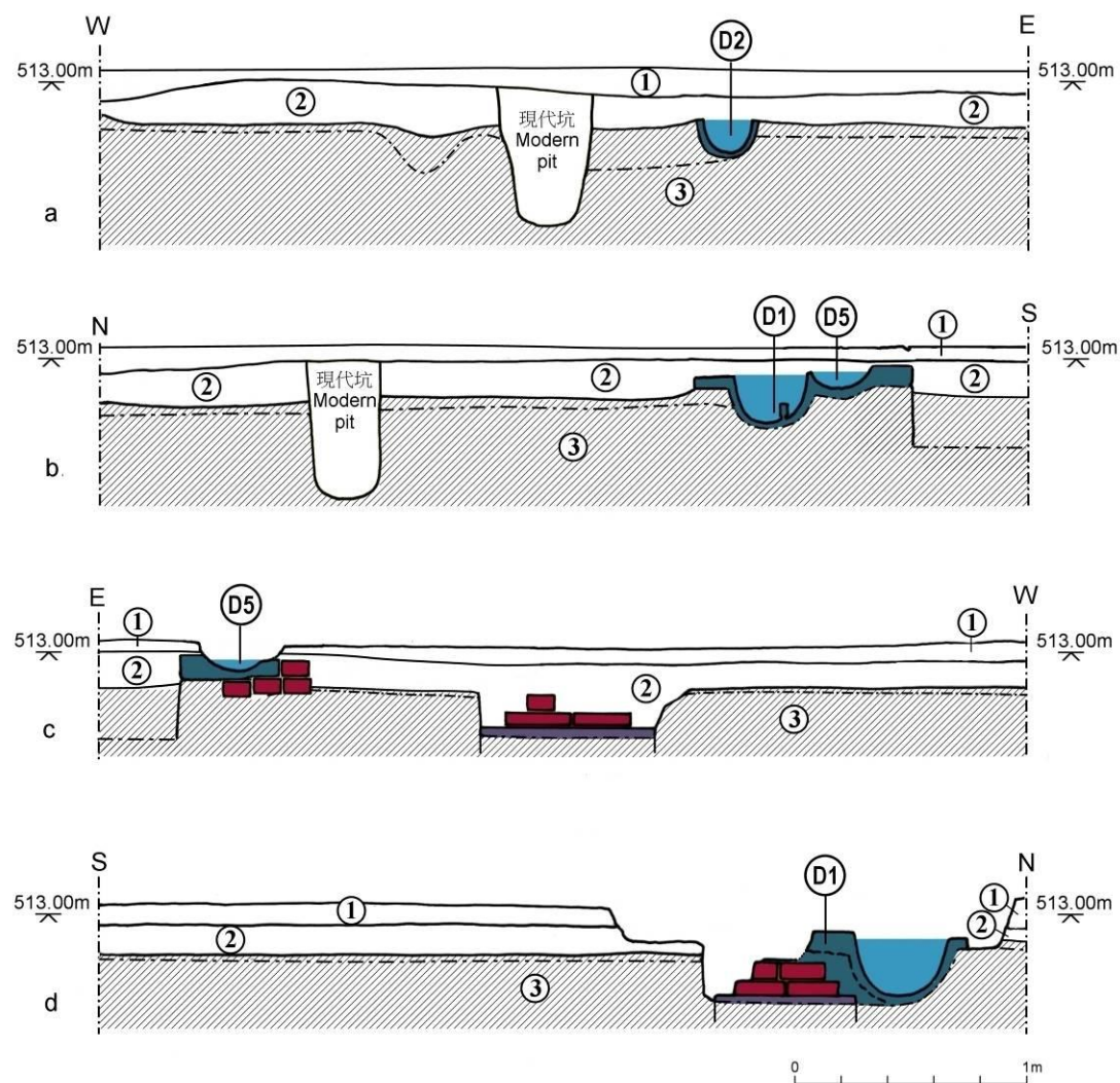
圖 6 探溝 TE 地層剖面圖 Fig 6 Profiles of test trench TE
