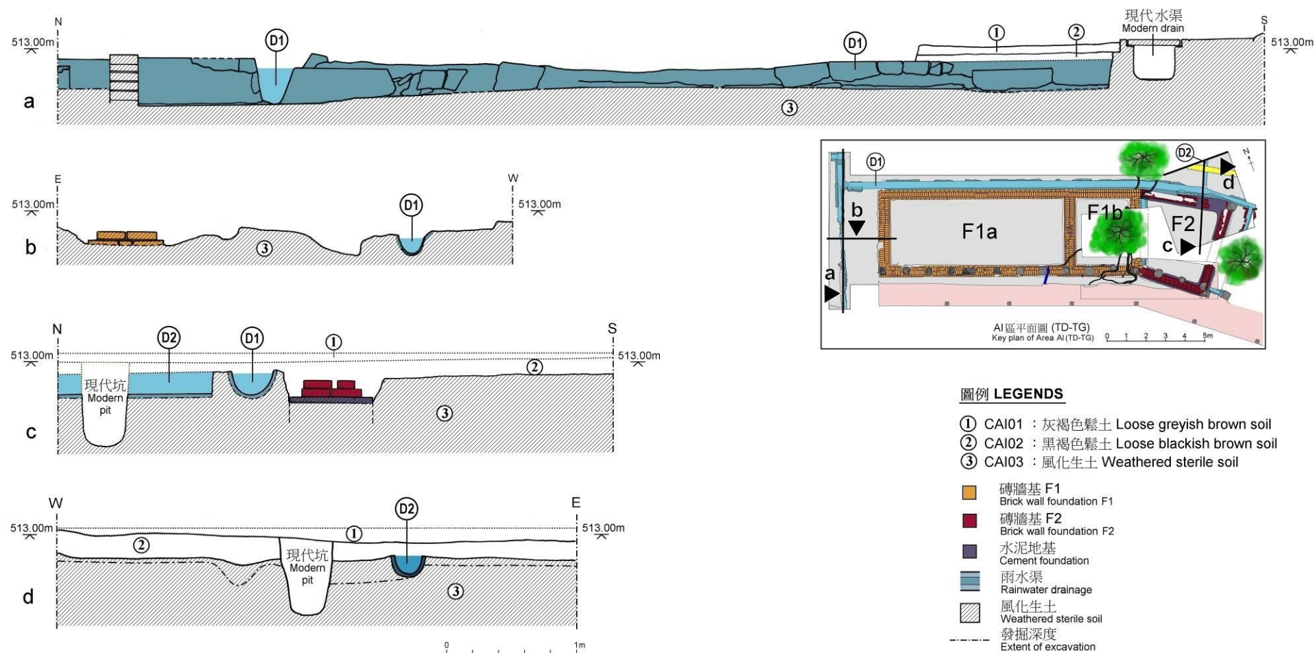
圖 11 雨水渠 D1, D2 剖面圖 Fig 11 Profiles of rainwater drainage D1 & D2
