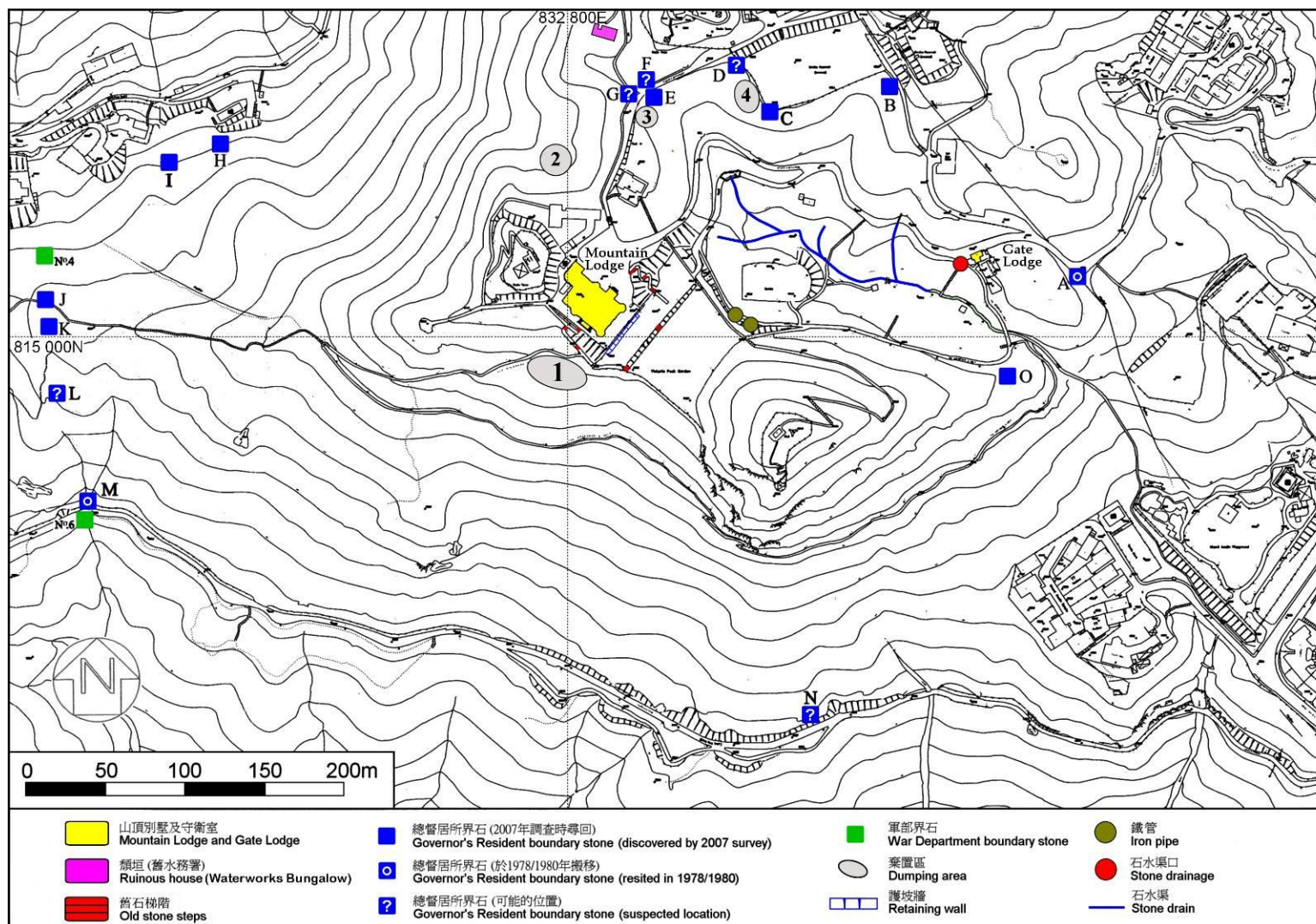
圖 55 2007 年考古調查發現的相關遺物 Fig 55 Remains identified by Archaeological Investigation, 2007
