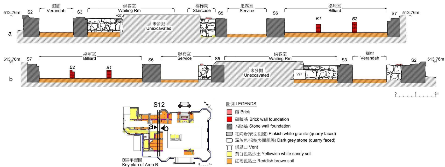
圖 44 石牆基 S12 側視圖 Fig 44 Side views of stone wall foundation S12
