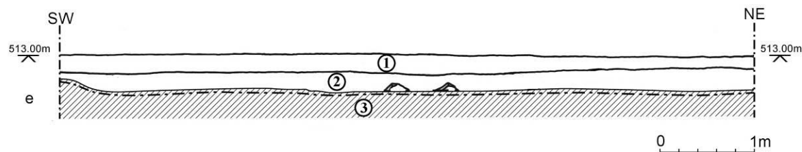
圖 14 探溝 TH 地層剖面圖 Fig 14 Profiles of test trench TH
