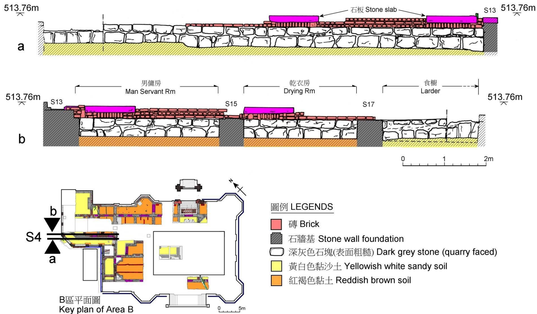
圖 36 石牆基 S4 側視圖 Fig 36 Side views of stone wall foundation S4
