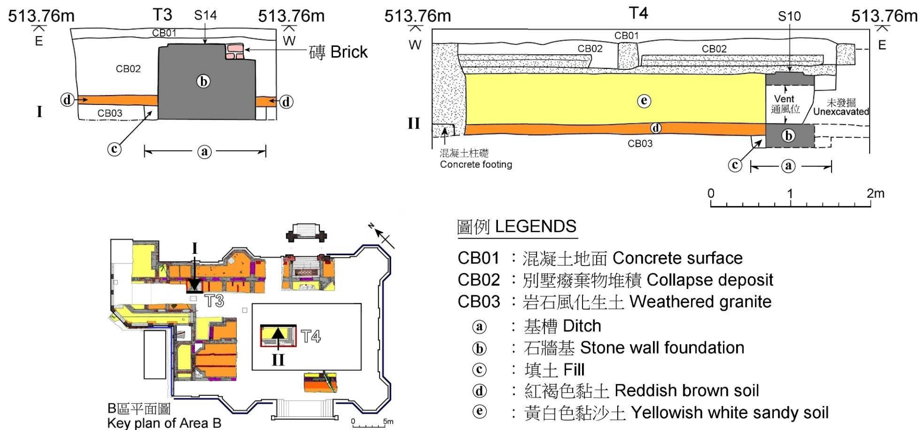
圖 20 探溝 T3 和 T4 地層剖面圖 Fig 20 Profiles of test trenches T3 and T4
