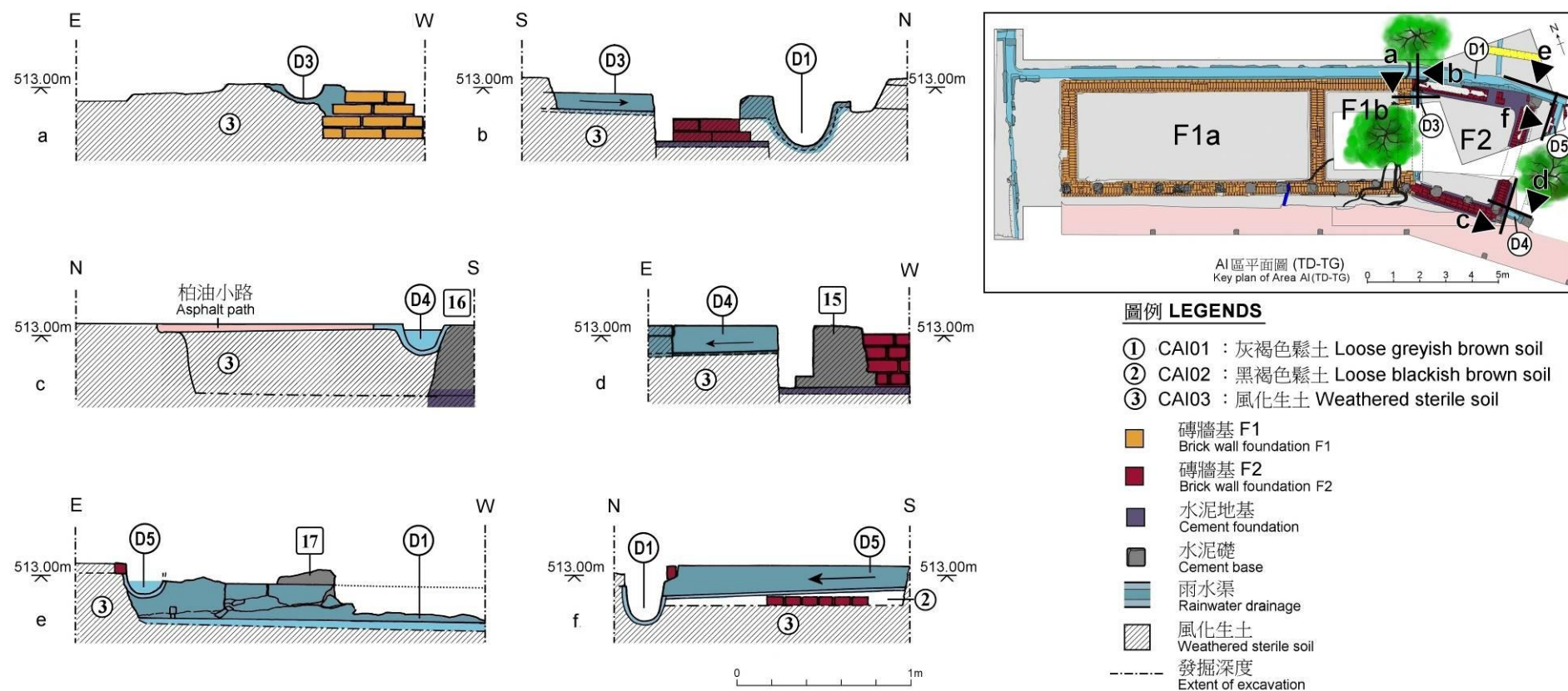
圖 12 雨水渠 D3, D4 和 D5 剖面圖 Fig 12 Profiles of rainwater drainage D3, D4 & D5
