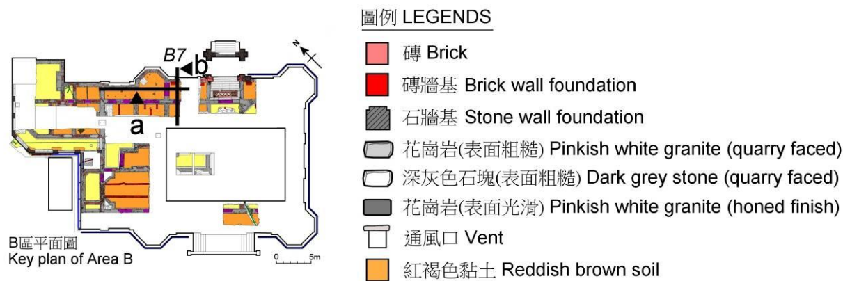
圖 53 磚牆基 B7 側視圖 Fig 53 Side views of brick wall foundation B7
