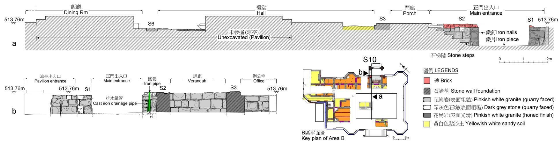
圖 42 石牆基 S10 側視圖 Fig 42 Side views of stone wall foundation S10
