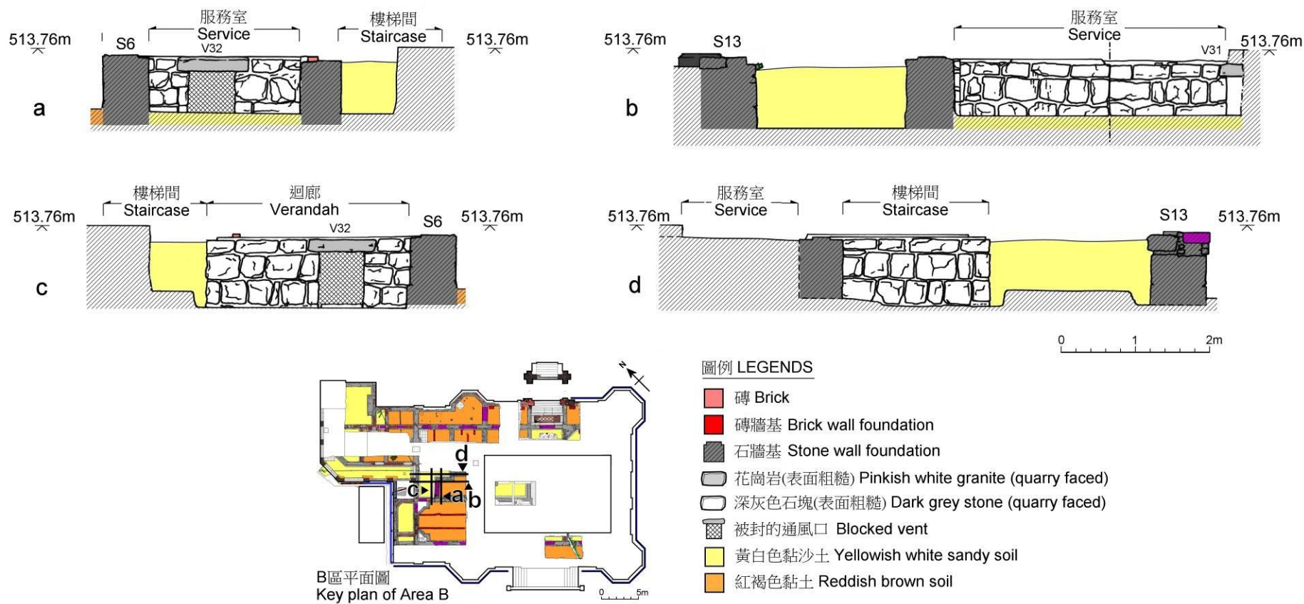
圖 37 石牆基 S5 側視圖 Fig 37 Side views of stone wall foundation S5
