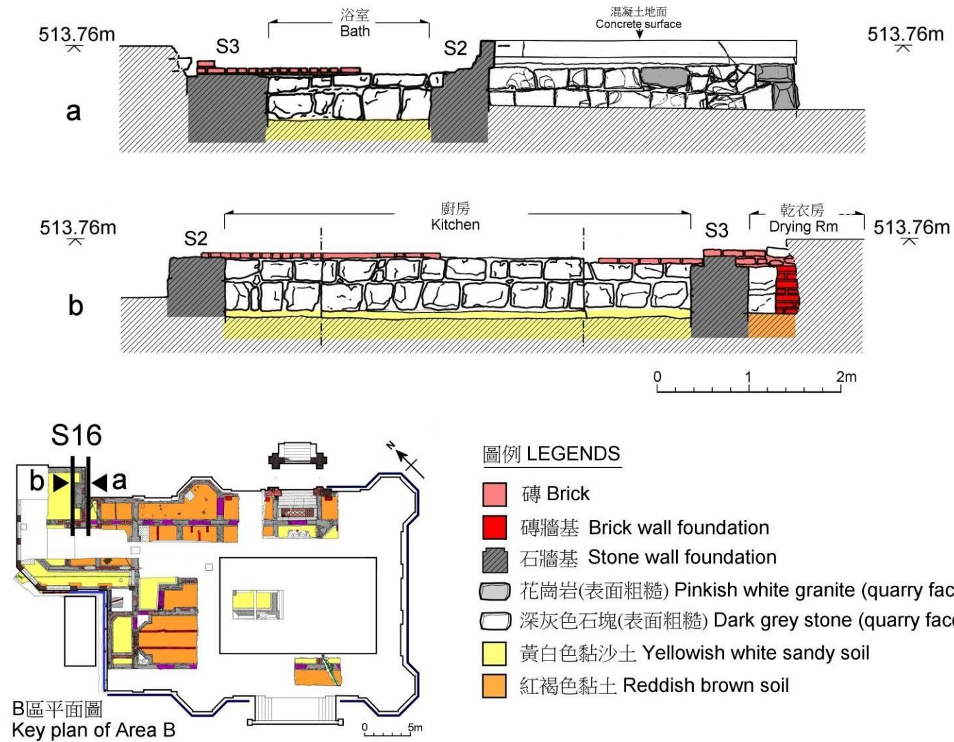
圖 48 石牆基 S16 側視圖 Fig 48 Side views of stone wall foundation S16
