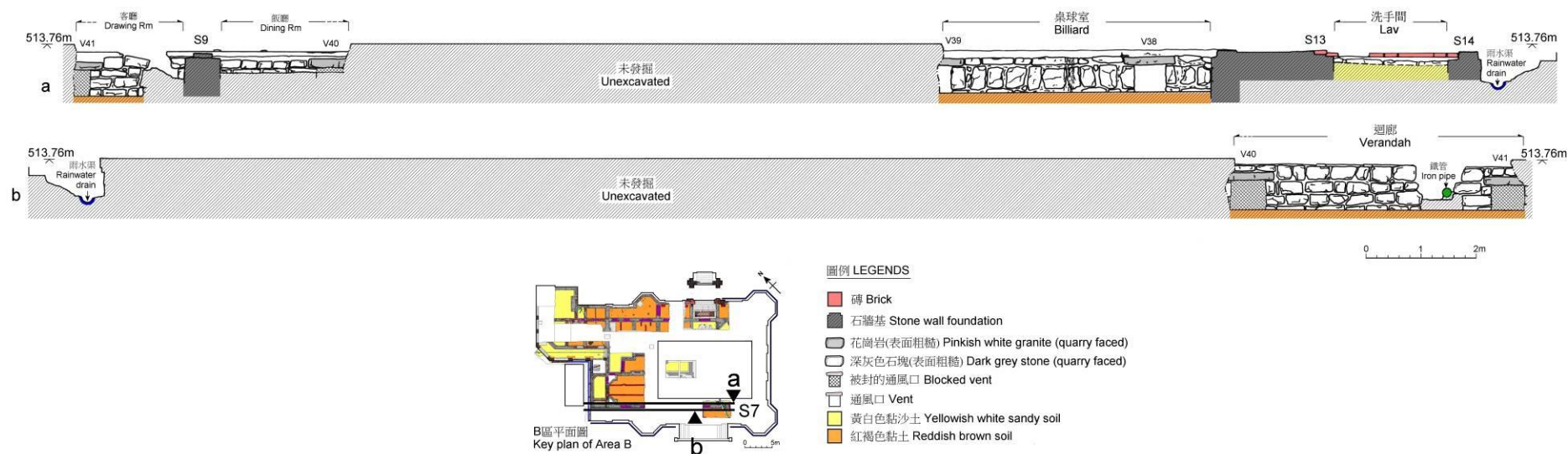
圖 39 石牆基 S7 側視圖 Fig 39 Side views of stone wall foundation S7
