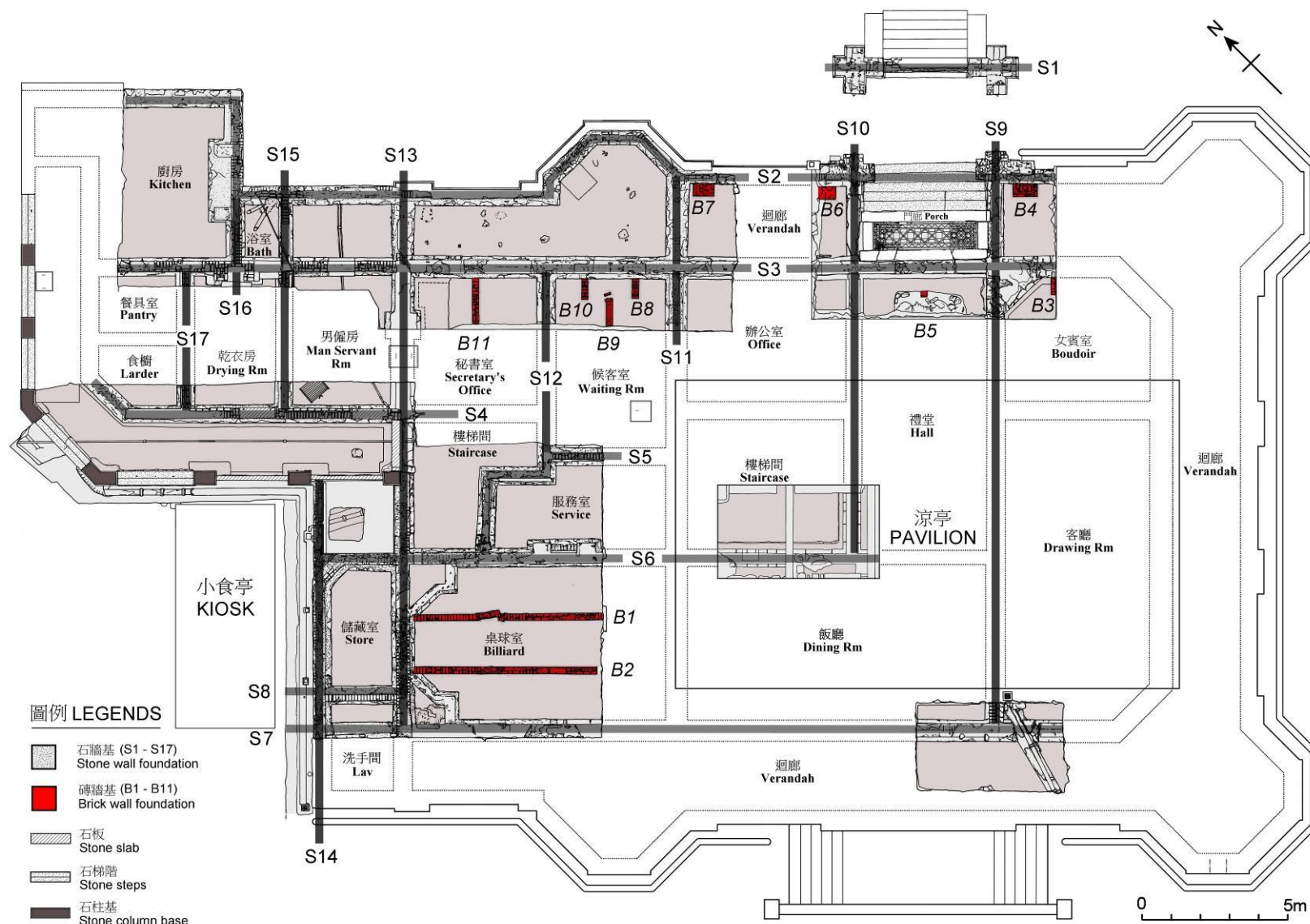
圖 24 B 區石牆基及磚牆基遺跡平面圖
