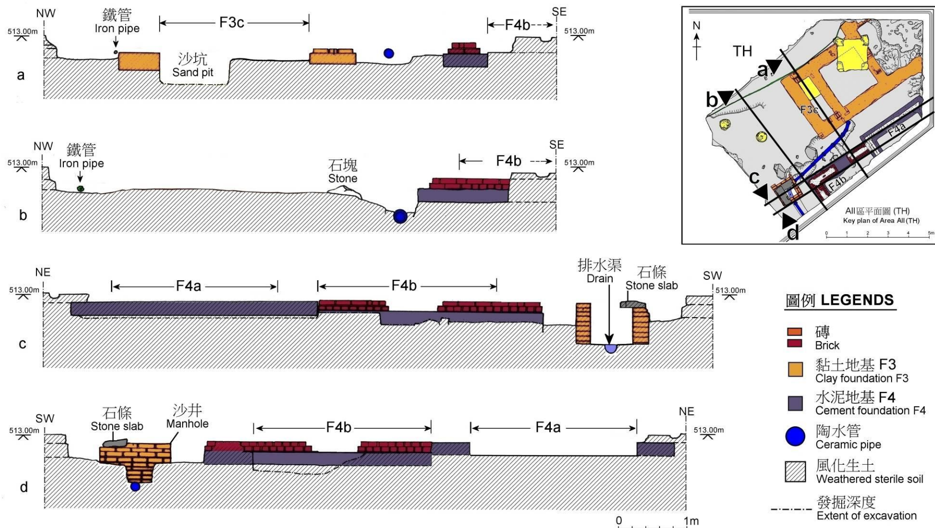
圖 17 磚牆基 F3 及 F4 剖面圖 (2) Fig 17 Profiles of brick wall foundation F3 & F4 (2)
