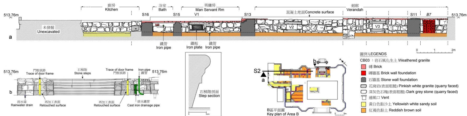
圖 34 石牆基 S2 側視圖 Fig 34 Side views of stone wall foundation S2
