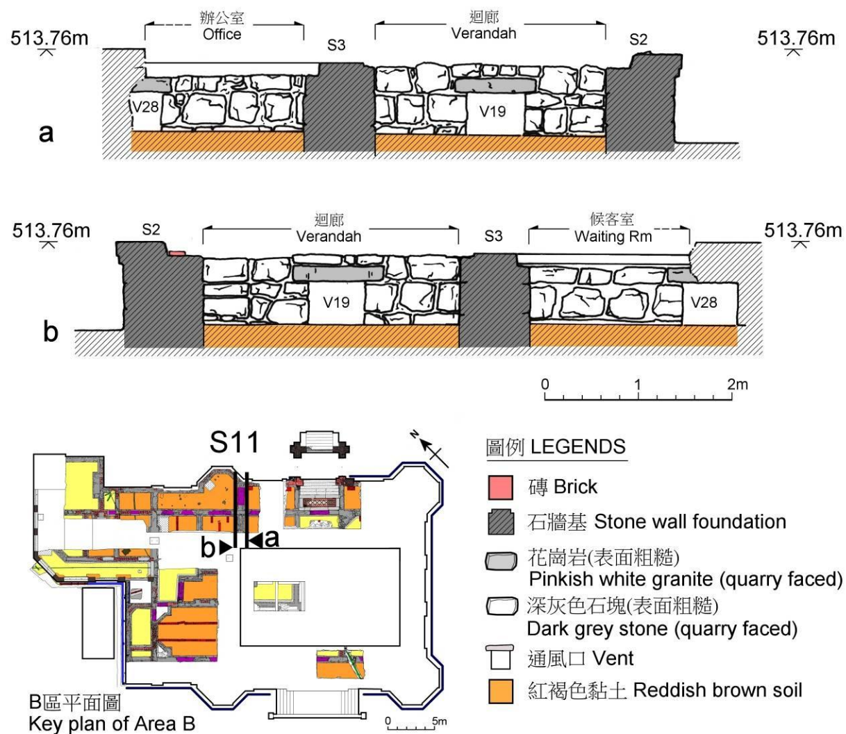
圖 43 石牆基 S11 側視圖 Fig 43 Side views of stone wall foundation S11
