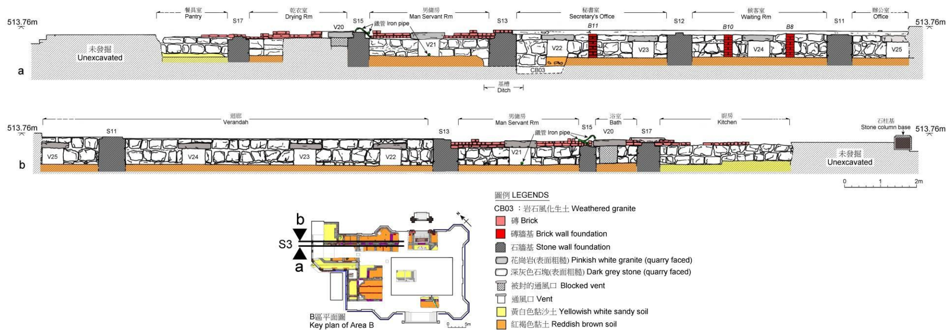
圖 35 石牆基 S3 側視圖 Fig 35 Side views of stone wall foundation S3
