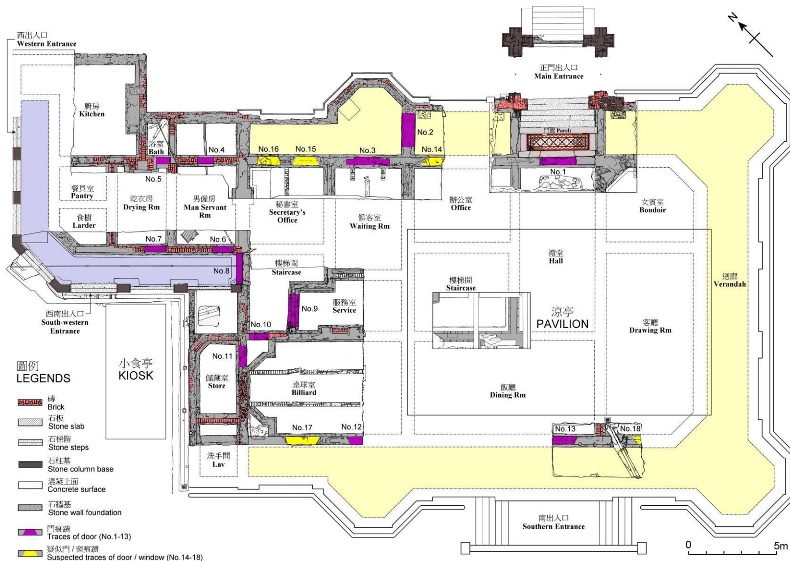
圖 26 B 區門窗痕跡平面圖
