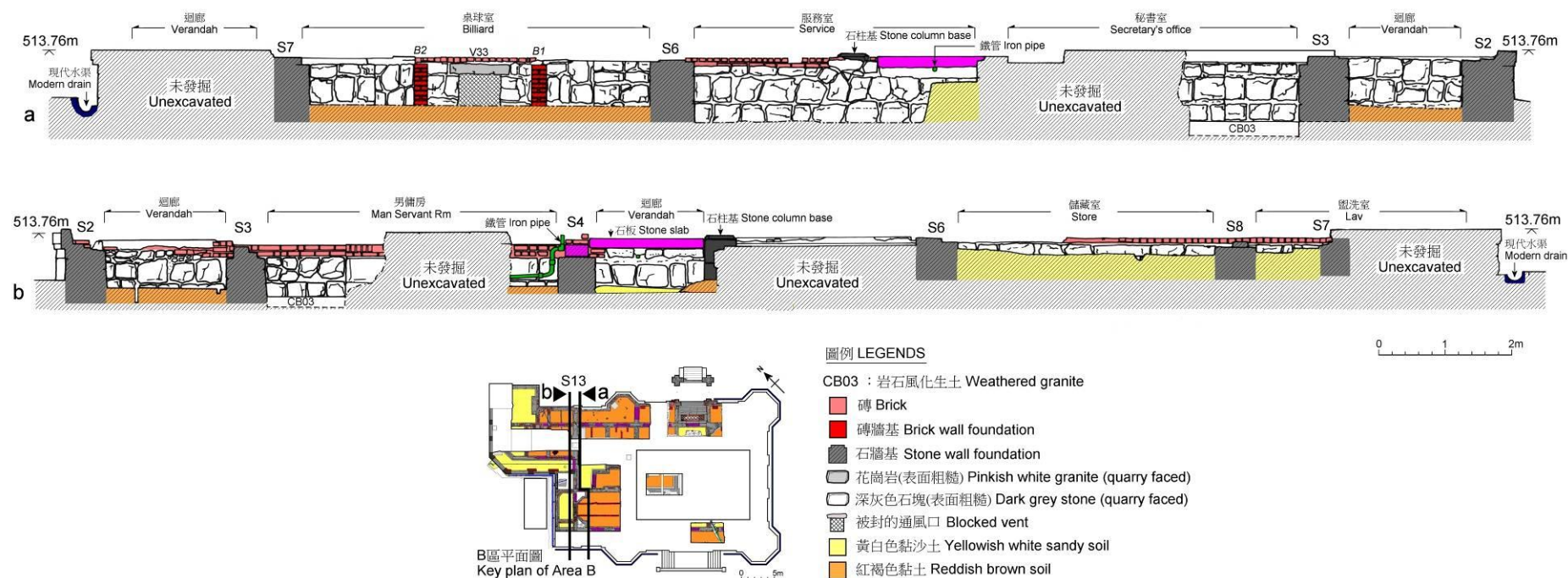
圖 45 石牆基 S13 側視圖 Fig 45 Side views of stone wall foundation S13
