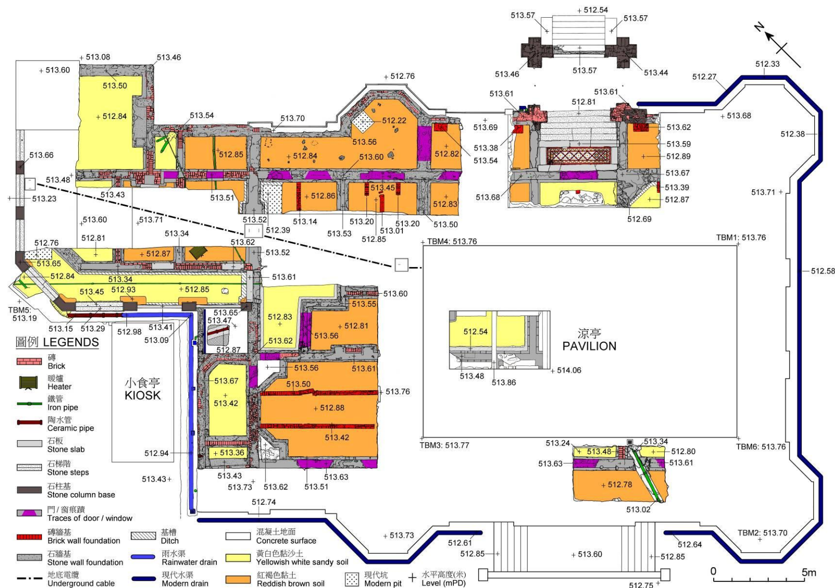
圖 22 B 區考古遺跡平面圖 Fig 22 Plan of features, Area B
