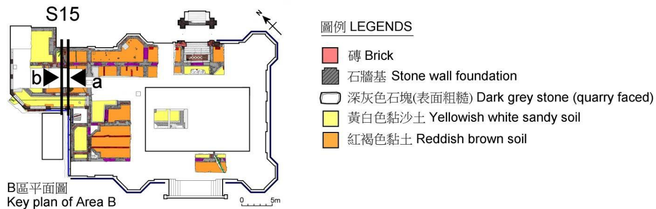
圖 47 B 區石牆基 S15 側視圖 Fig 47 Side views of stone wall foundation S15
