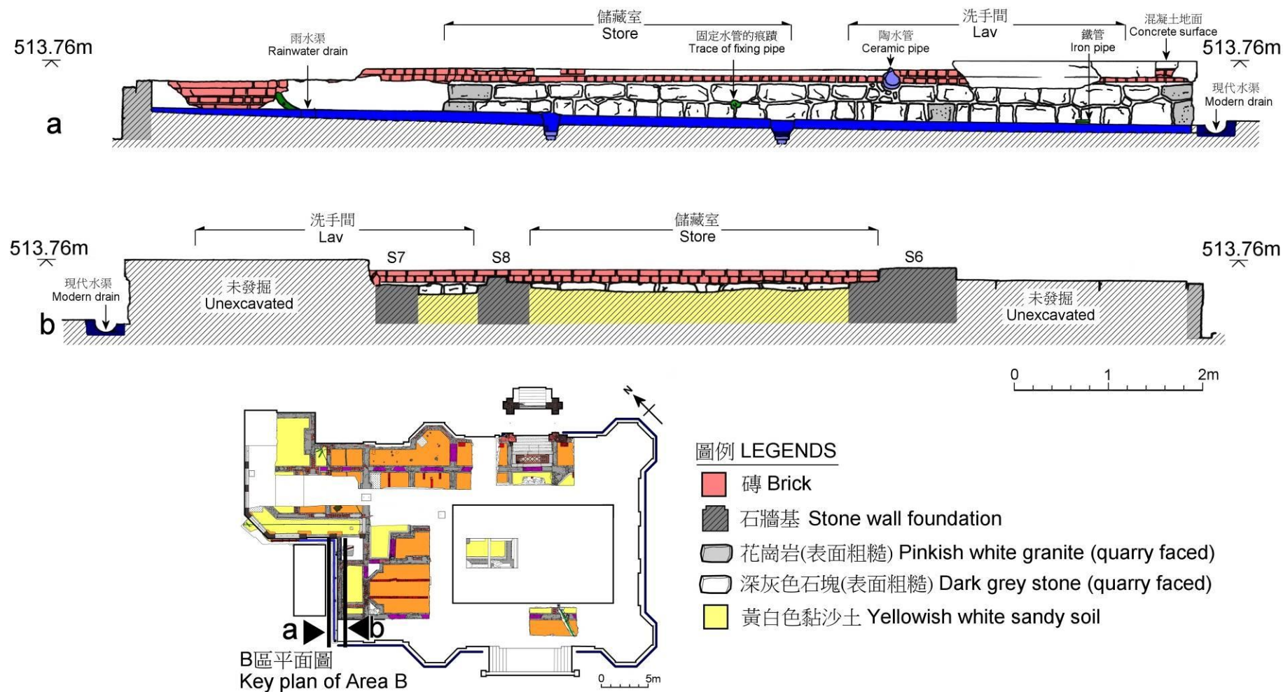
圖 46 B 區石牆基 S14 側視圖 Fig 46 Side views of stone wall foundation S14
