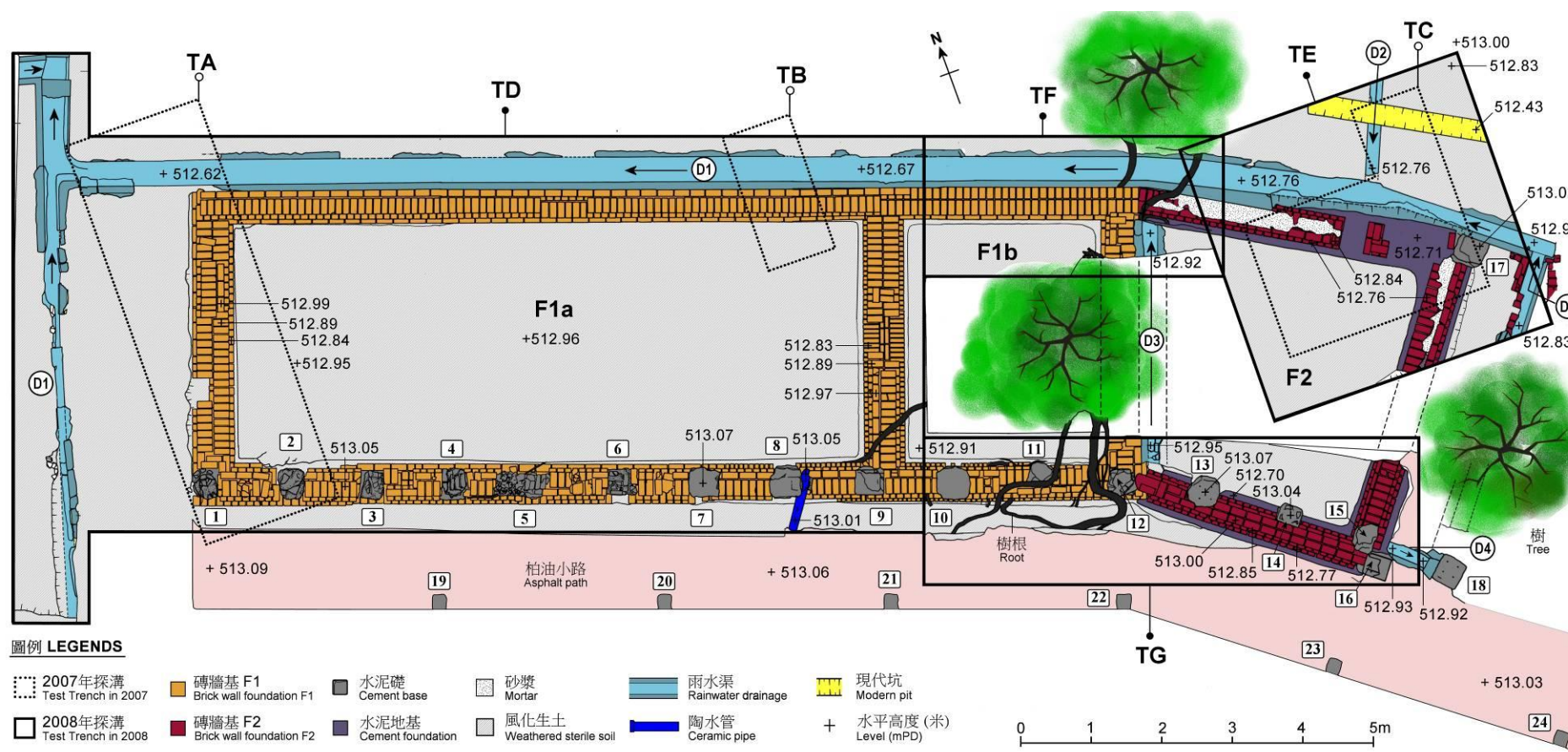
圖 4 AI 區平面圖 Fig 4 Plan of Area AI
