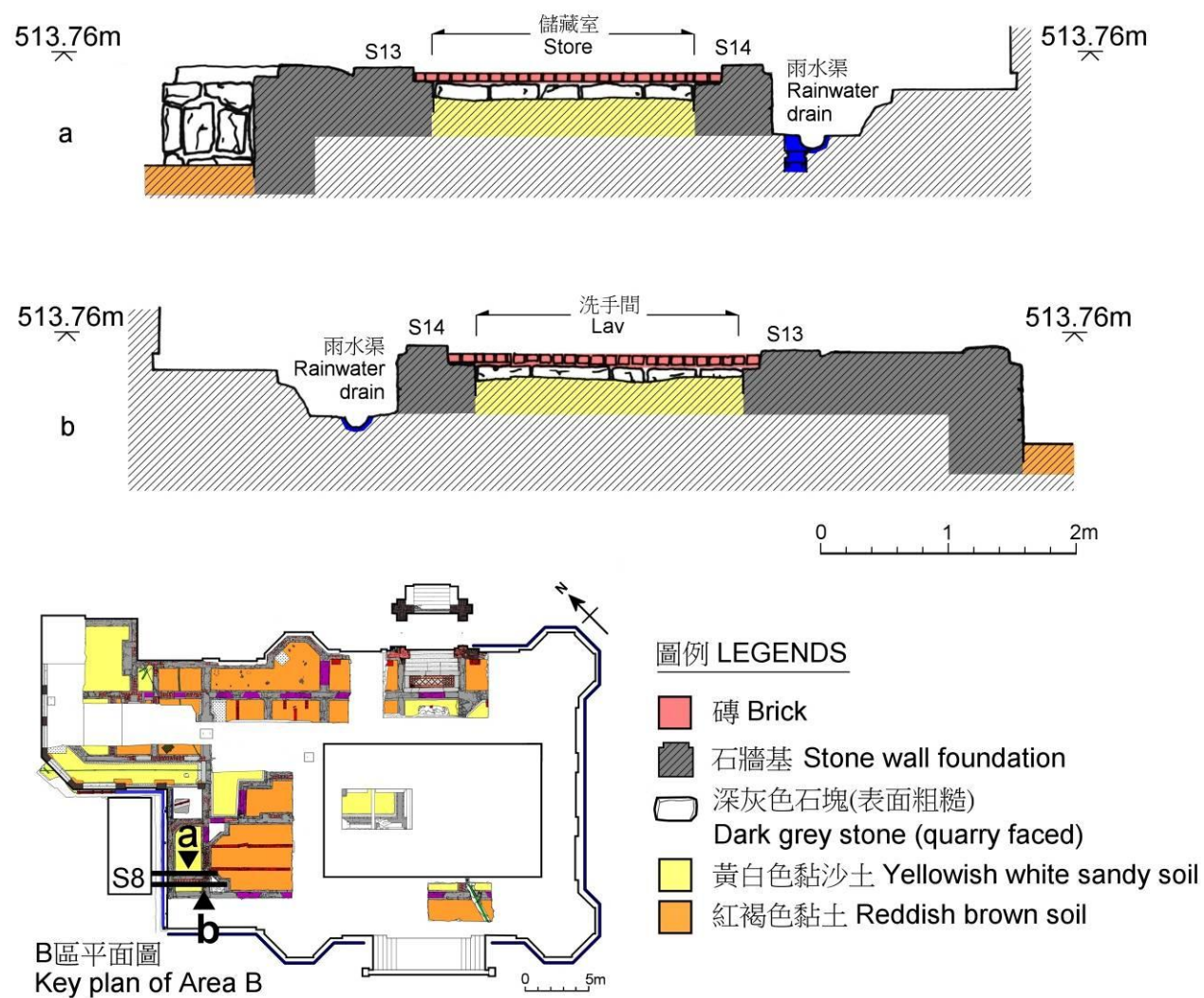
圖 40 石牆基 S8 側視圖 Fig 40 Side views of stone wall foundation S8
