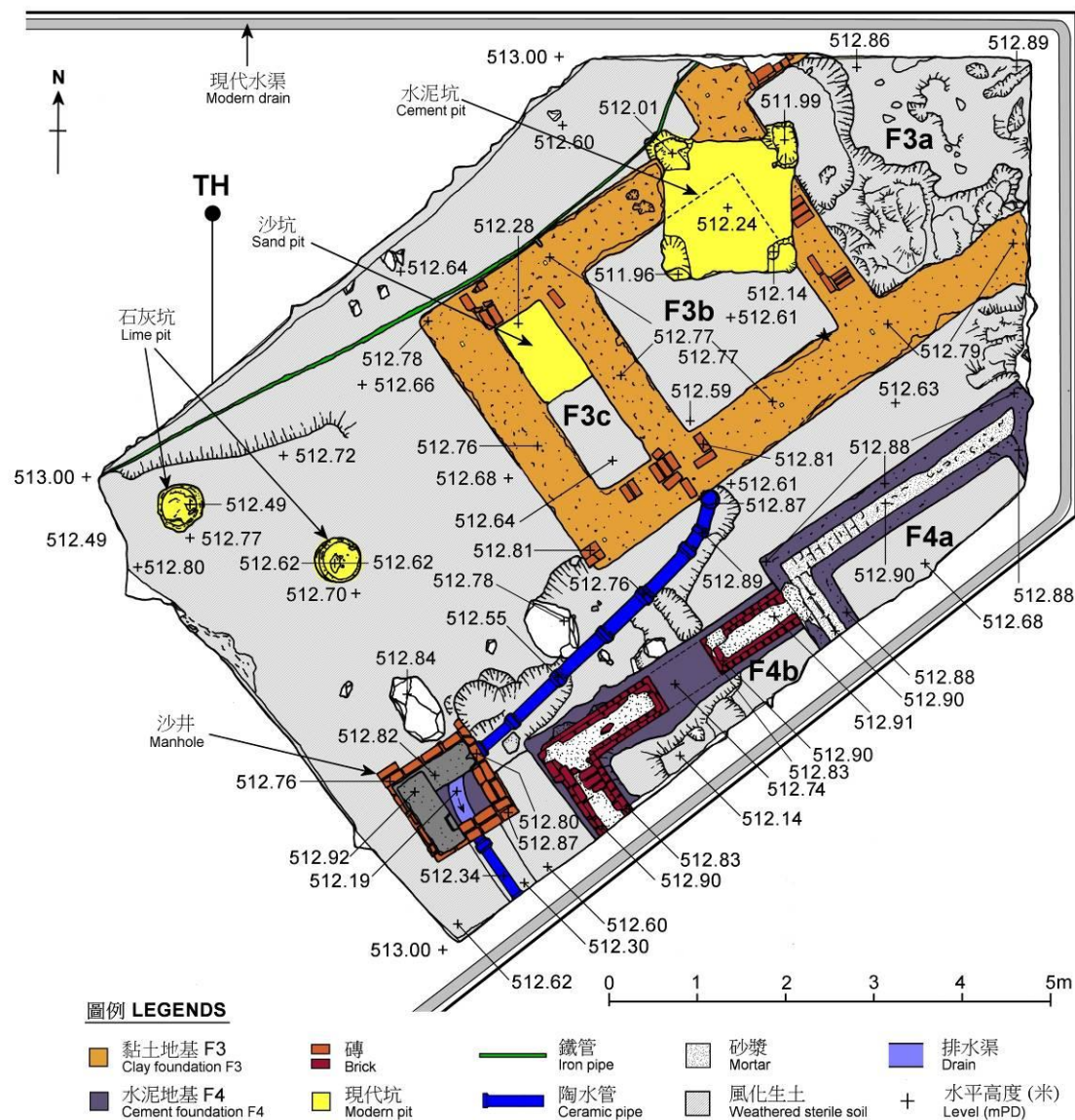
圖 13 AII 區平面圖 Fig 13 Plan of Area AII
