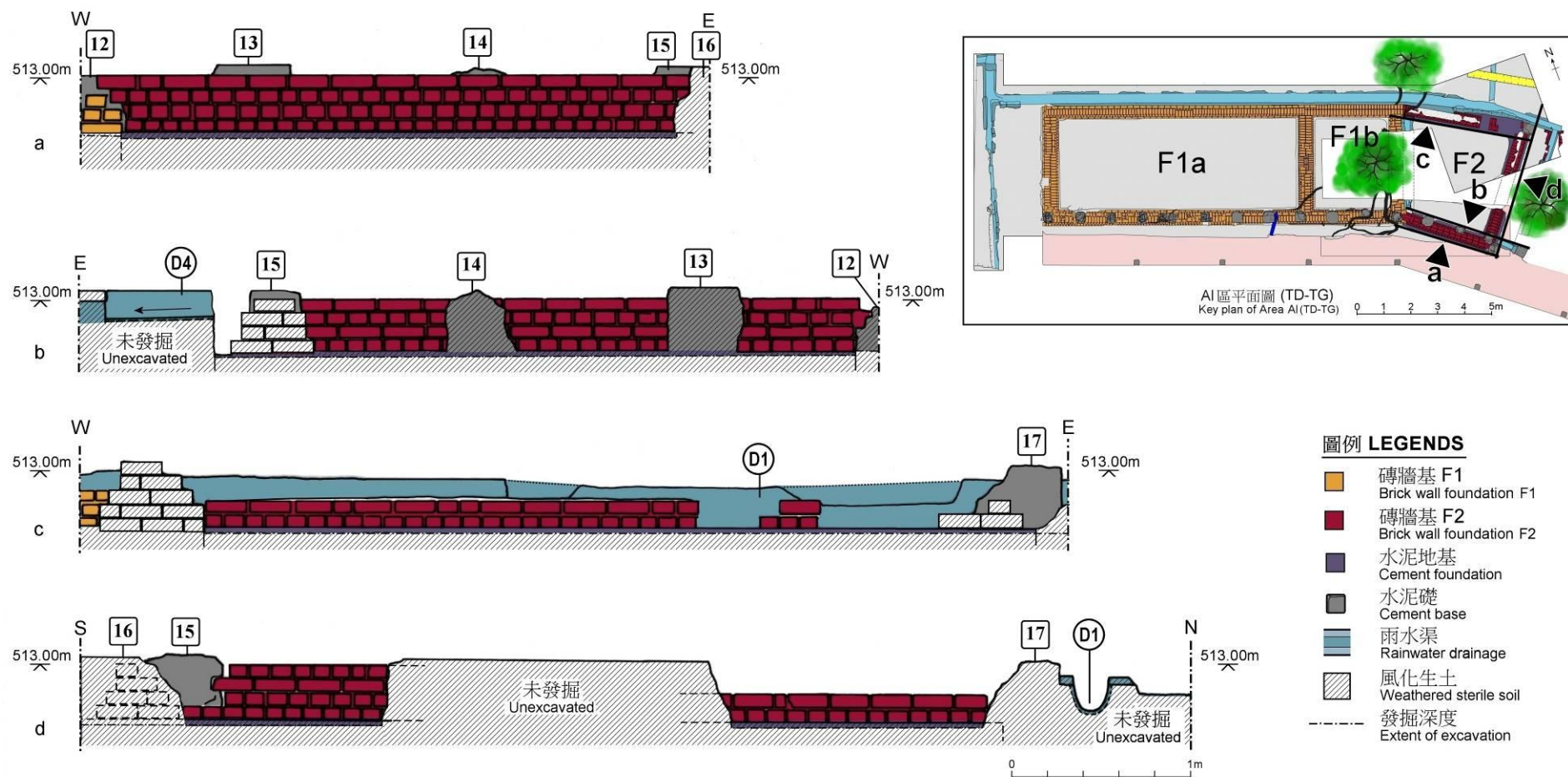
圖 10 磚牆基 F2 側視圖 Fig 10 Side views of brick wall foundation F2
