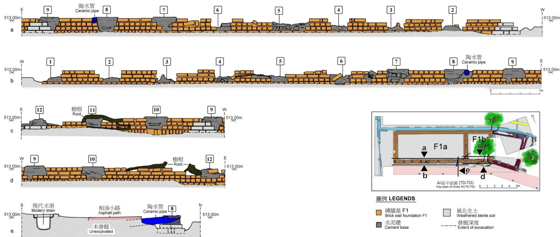
圖 8 磚牆基 F1 側視圖 (1) Fig 8 Side views of brick wall foundation F1 (1)
