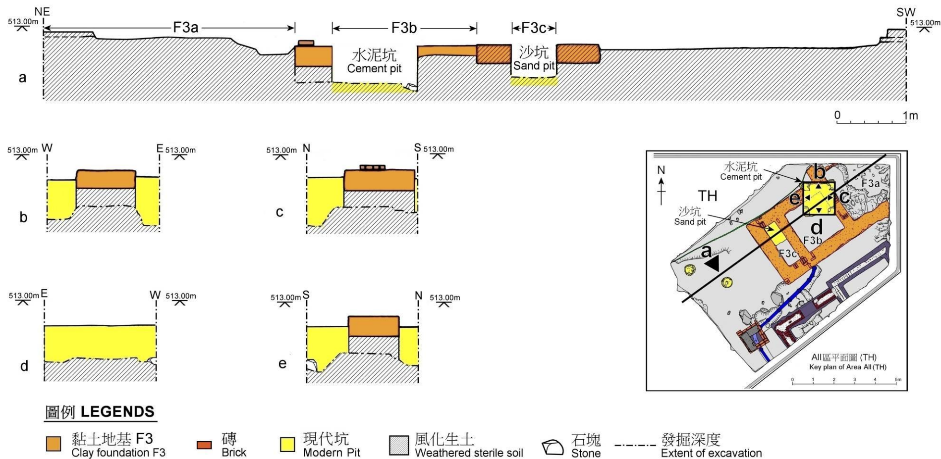
圖 15 磚牆基 F3 及現代坑剖面圖 Fig 15 Profiles of brick wall foundation F3 & modern pit
