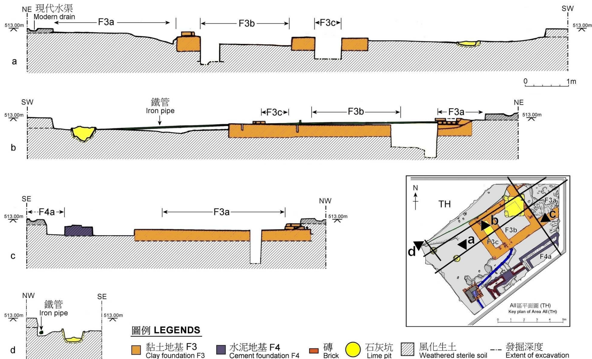
圖 16 磚牆基 F3 及 F4 側視剖面圖 (1) Fig 16 Profiles of brick wall foundation F3 & F4 (1)
