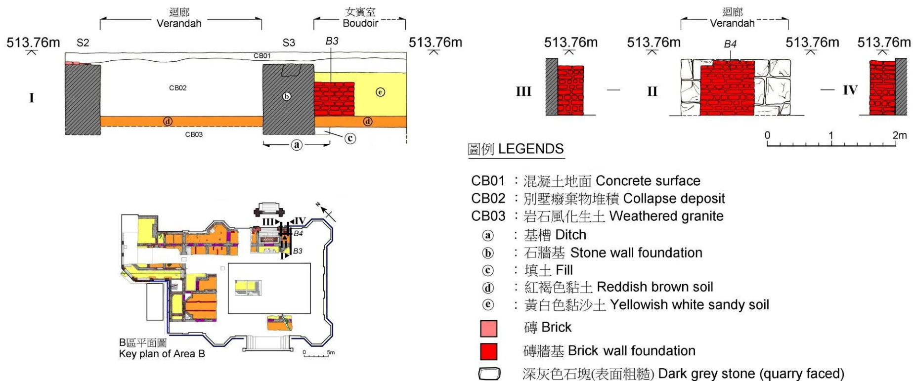
圖 51 磚牆基 B3 及 B4 側視圖 Fig 51 Side views of brick wall foundations B3 and B4
