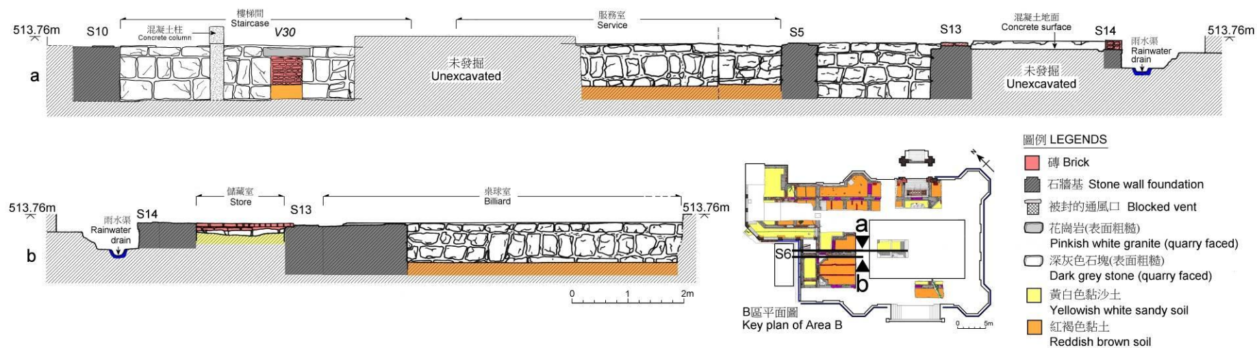
圖 38 石牆基 S6 側視圖 Fig 38 Side views of stone wall foundation S6
