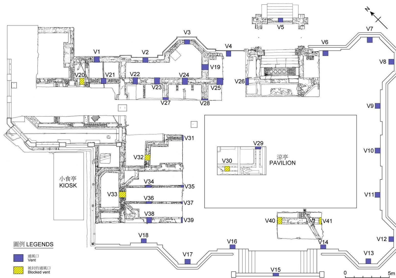
圖 25 B 區通風口平面圖 Fig 25 Plan of vents, Area B
