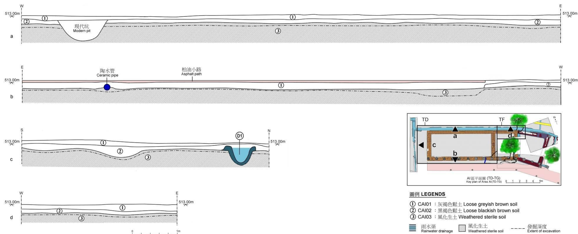
圖 5 探溝 TD，TF 地層剖面圖 Fig 5 Profiles of test trenches TD and TF
