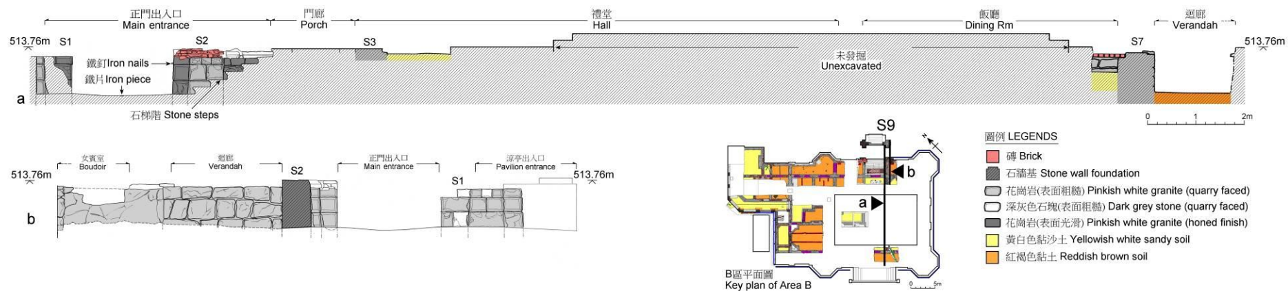
圖 41 石牆基 S9 側視圖 Fig 41 Side views of stone wall foundation S9
